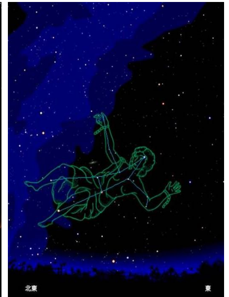
アンドロメダ座（星図より）
